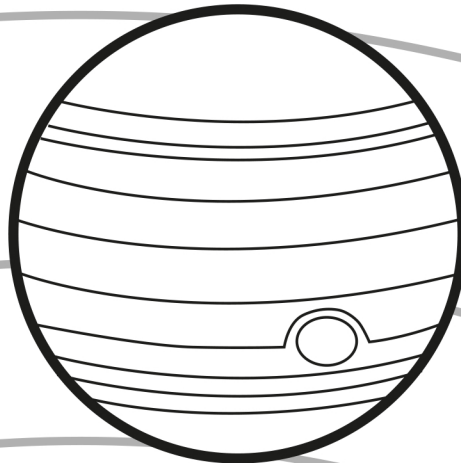
مشتری Jupiter
