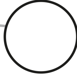
اورانوس Uranus
